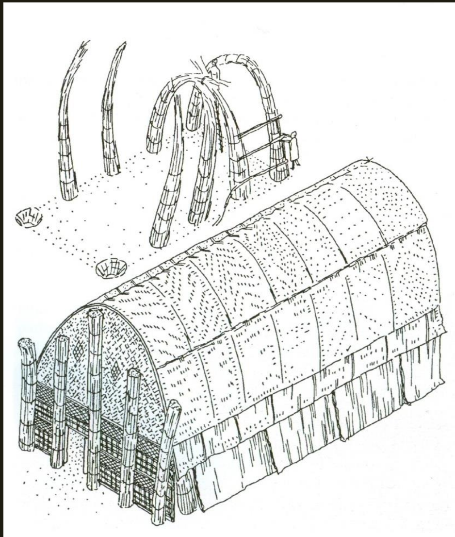
Nád-ház / Mudhif / Irak / A Madanok (Ma'dan, mocsári arab) lakó- és közösségi épülete
